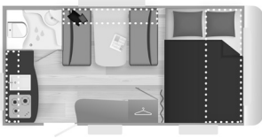
ANTARÈS STYLE 400 • 4,20 x 1,95 m
