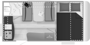
ALBA 400 • 4,20 x 1,95 m
