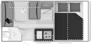
ALBA 390 • 4,00 x 1,95 m
