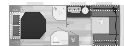
ALLEGRA OPTIMA 560 • 5,80 x 2,15 m
