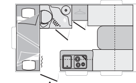
ANTARÈS 386 • 3,80 x 2,15 m
